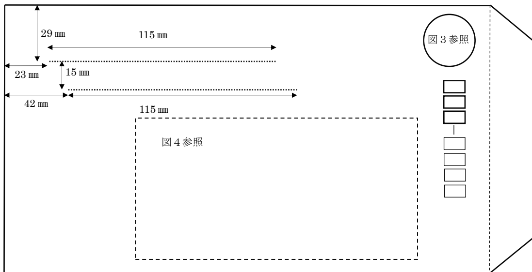
図 1（長形 3 号表面）
