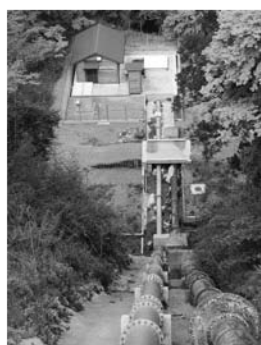
面白峠の小水力発電所
