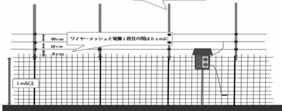
【参考】サル用複合柵の設置例
